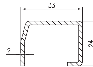
Art.-Nr. 623500 Flügelverstärkung 2 mm ST, t = 2 mm I_x = 1,05 \text{ cm}^4 I_y = 2,54 \text{ cm}^4
